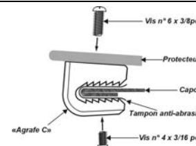
Illustration n°3: Configuration de l'agrafe
