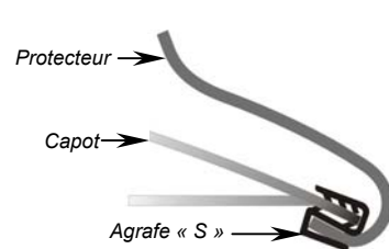
Illustration n°2: Emplacement d'agrafe «S» le capot
