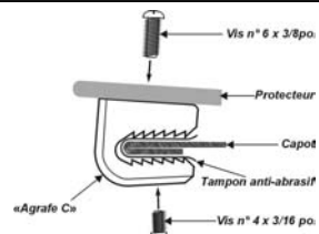
Illustration n°3: Configuration de l'agrafe
