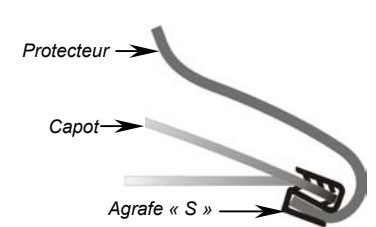
Illustration n°2: Emplacement d'agrafe «S» le capot
