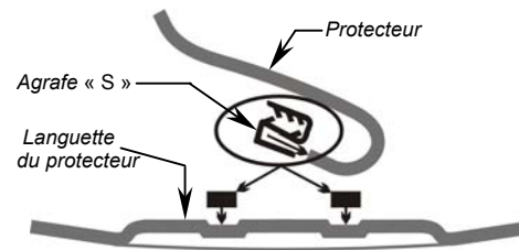
Illustration n°3: Configuration de l'agrafe
