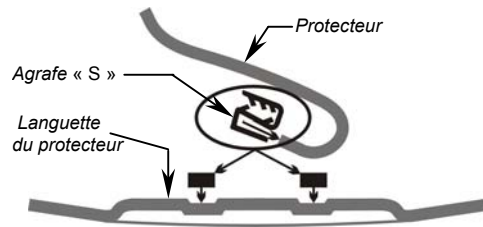
Illustration n°3: Configuration de l'agrafe
